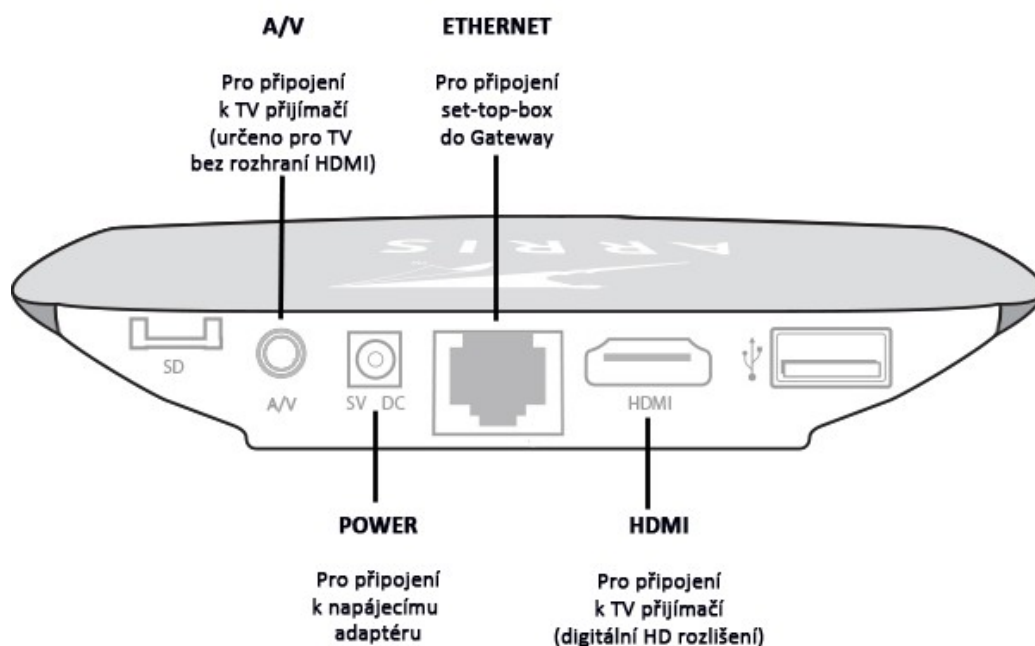
Obr. 1: Zobrazenie a popis portov na zadnom paneli set-top-boxu
